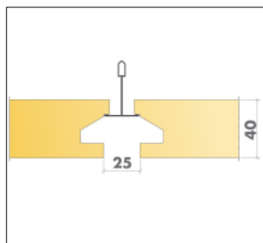
Undertaksplatta Master Eg i profil i ett T24 bärverk.
