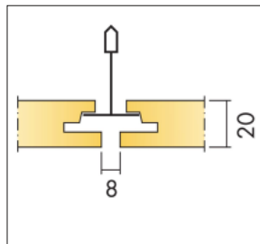
Undertaksplatta Focus E i profil i ett T24 bärverk.
