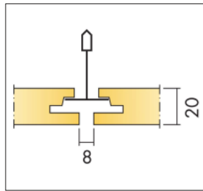
Undertaksplatta Focus Dg i profil i ett T24 bärverk.
