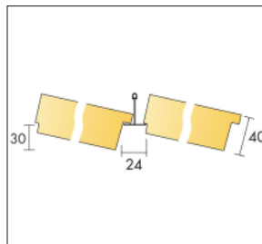
Undertaksplatta Focus Ez i profil i ett T24 bärverk.
