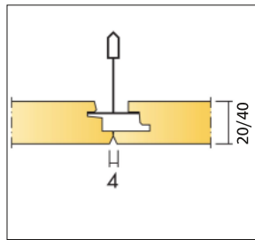
Undertaksplatta Focus Ds i profil i ett T24 bärverk.
